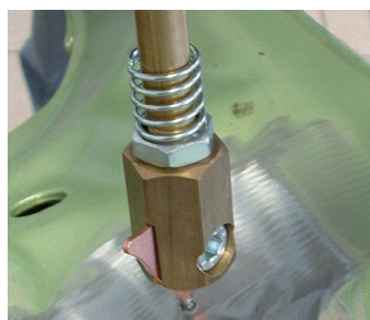
Soldadura por puntos de las arandelas especiales
