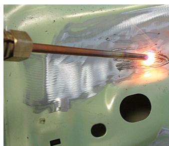
Calentado de las planchas
