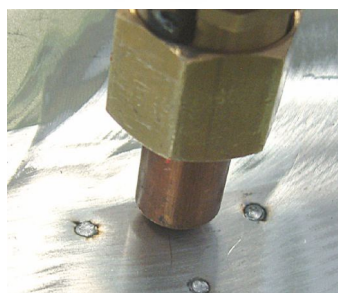
Achatado de las bulas
