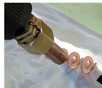
Soldadura por puntos de las arandelas
